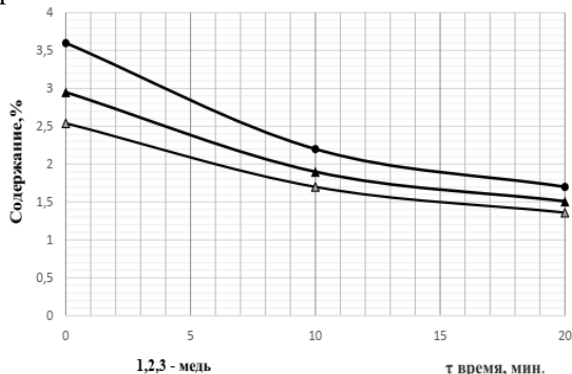
Рис. 2. Остаточное содержание меди в конвертерном шлаке при его восстановлении клинкером
