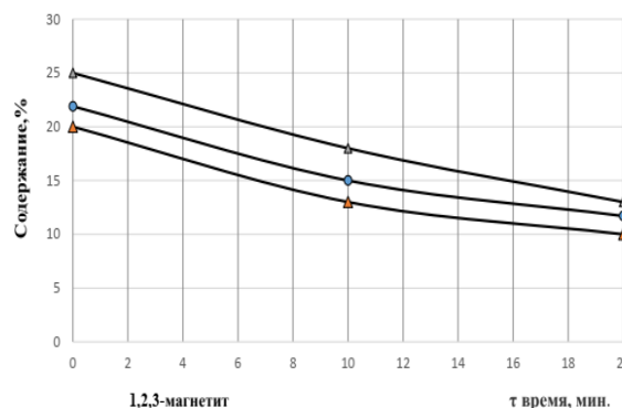
Рис. 1. Остаточное содержание магнетита конвертерного шлака при восстановлении его клинкером
